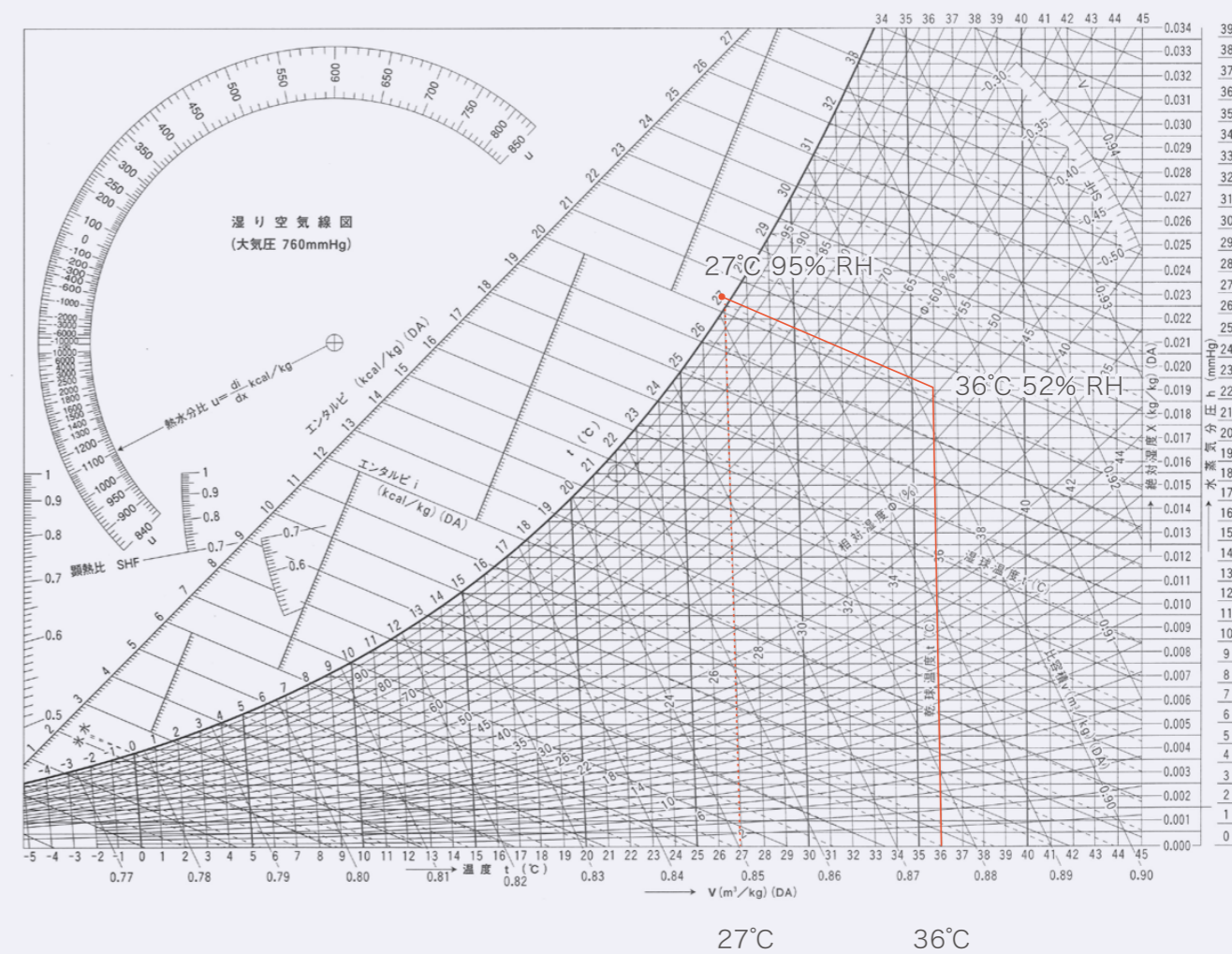
湿り空気線図
